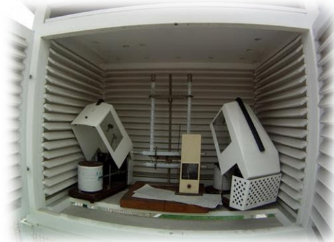
Wnętrze klatki meteorologicznej
